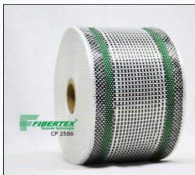
CP- 2586 Green Espessura: 0,30mm Largura: 80mm Comprimento do rolo: 50m
