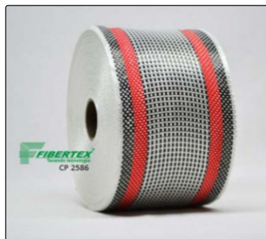
CP- 2586 Red Espessura: 0,30mm Largura: 80mm Comprimento do rolo: 50m
