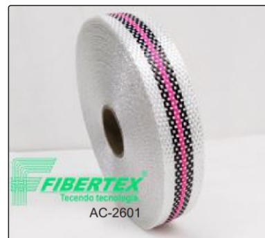
AC- 2601 Espessura: 0,25mm Largura: 25mm Comprimento do rolo: 50m
