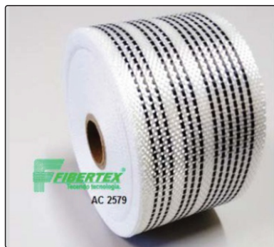
AC- 2579 Espessura: 0,25mm Width: 80mm Length: 50m
