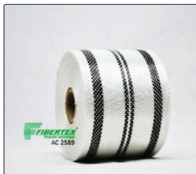
AC- 2589 Espessura 0,25mm Largura: 80mm Comprimento do rolo: 50m
