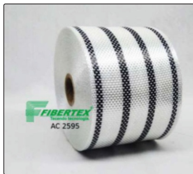
AC- 2595 Espessura: 0,25mm Largura: 80mm Comprimento do rolo: 50m
