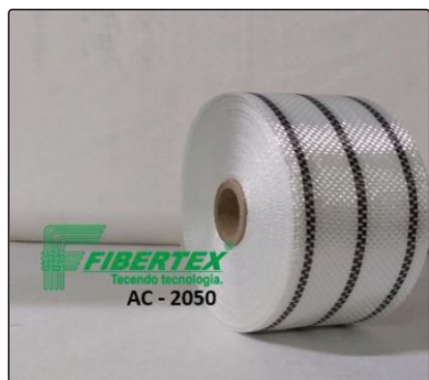
AC- 2050 Espessura: 0,20mm Width: 50mm Length: 50m
