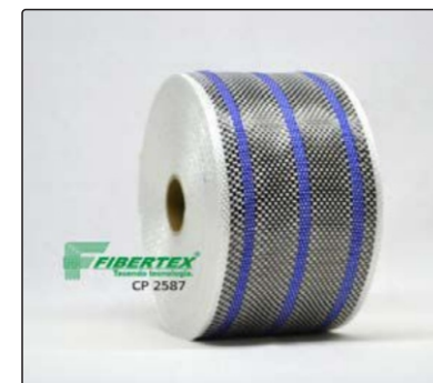
CP - 2587 Blue Espessura: 0,45mm Largura: 75mm Comprimento do rolo: 50m
