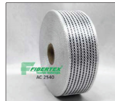
AC- 2540 Espessura: 0,25mm Width: 40mm Length: 50mm
