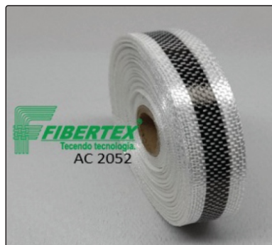
AC- 2052 Espessura: 0,20mm Width: 25mm Length: 50m
