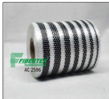
AC- 2596 Espessura: 0,25mm Largura: 100mm Comprimento do rolo: 50m
