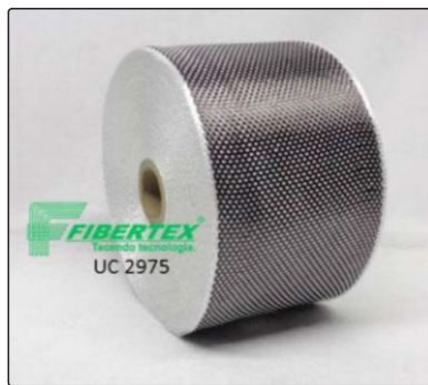
UC - 2975 Espessura: 0,45mm Largura: 75mm Comprimento do rolo: 50m
