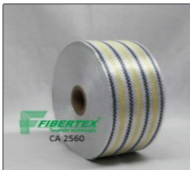
AC- 2560 Espessura: 0,25mm Largura: 60mm Comprimento do rolo: 50m
