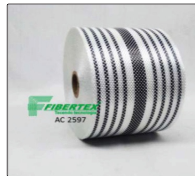
AC- 2597 Espessura: 0,25mm Largura: 80mm Comprimento do rolo: 50m
