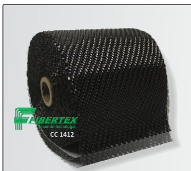
CC - 1412 Espessura: 1,40mm Largura: 120mm Comprimento do Rolo: 50m
