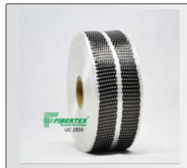
UC- 2850 Espessura: 0,45mm Largura: 50mm Comprimento do rolo: 50m
