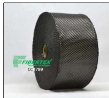
CC - 4799 Espessura: 0,47mm Largura: 100mm Comprimento do rolo: 50m
