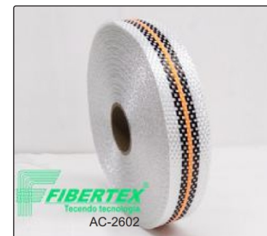
AC- 2602 Espessura: 0,25mm Largura: 25mm Comprimento do rolo: 50mm
