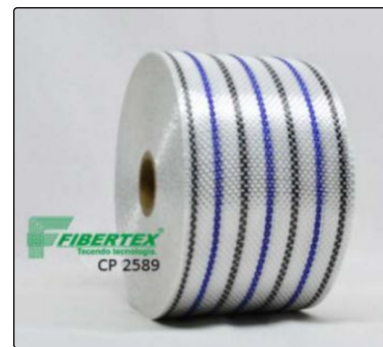
CP - 2589 Blue Espessura: 0,35mm Largura: 80mm Comprimento do rolo: 50m
