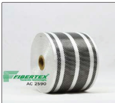
AC- 2590 Espessura: 0,25mm Largura: 75mm Comprimento do rolo: 50m
