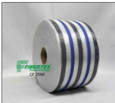
CP - 2590 Blue Espessura: 0,35mm Largura: 80mm Comprimento do rolo: 50m
