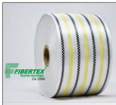
AC- 2580 Espessura: 0,25mm Largura: 80mm Comprimento do rolo: 50m
