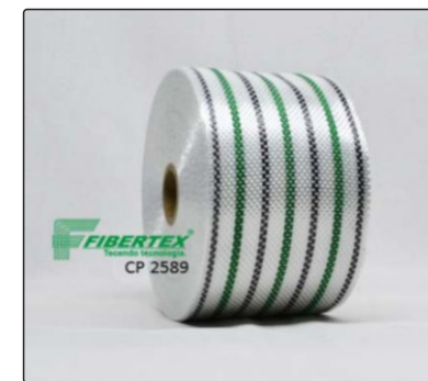
CP - 2589 Green Espessura: 0,35mm Largura: 80mm Comprimento do rolo: 50m
