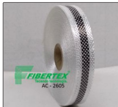
AC- 2605 Espessura: 0,25mm Largura: 22mm Comprimento do rolo: 50m
