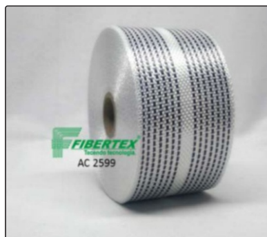
AC- 2599 Espessura: 0,25mm Largura: 70mm Comprimento do rolo: 50m
