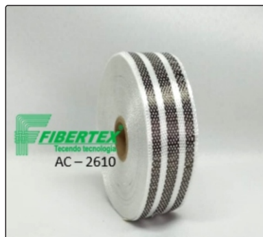
AC- 2610 Espessura: 0,20mm Largura: 47mm Comprimento do rolo: 50m
