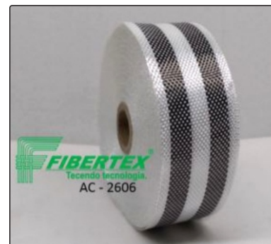
AC- 2606 Espessura: 0,25mm Largura: 45mm Comprimento do rolo: 50m
