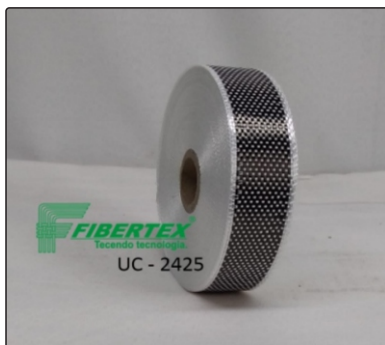
UC - 2425 Espessura: 0,24mm Largura: 25mm Comprimento do rolo: 50m
