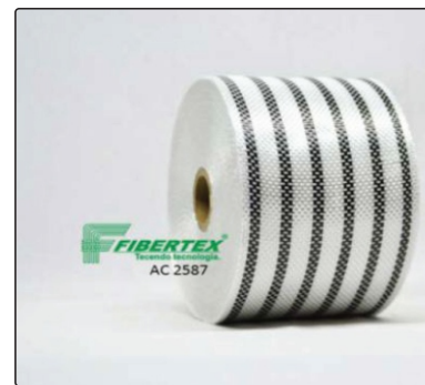
AC- 2587 Espessura 0,25mm Largura: 80mm Comprimento do rolo: 50m
