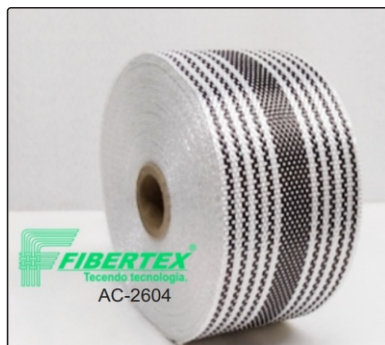
AC- 2604 Espessura: 0,25mm Largura: 65mm Comprimento do rolo: 50m
