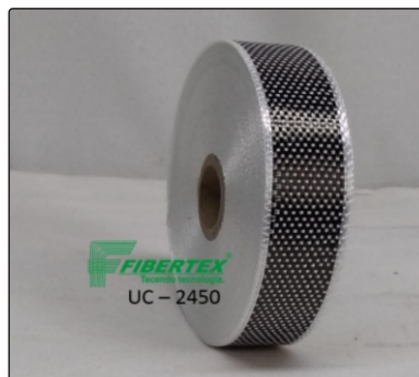
UC - 2450 Espessura: 0,24mm Largura: 50mm Comprimento do rolo: 50m
