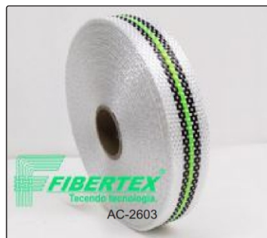
AC- 2603 Espessura: 0,25mm Largura: 25mm Comprimento do rolo: 50m
