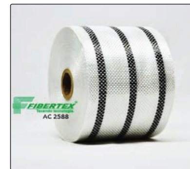
AC- 2588 Espessura 0,25mm Largura: 80mm Comprimento do rolo: 50m
