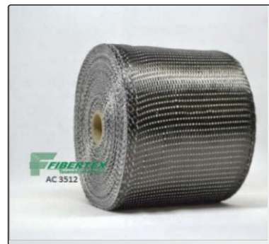
AC - 3512 Espessura: 0,35mm Largura: 120mm Comprimento do rolo: 50m
