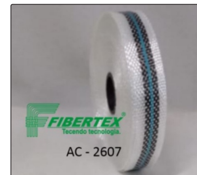
AC- 2607 Espessura: 0,25mm Largura: 25mm Comprimento do rolo: 50m
