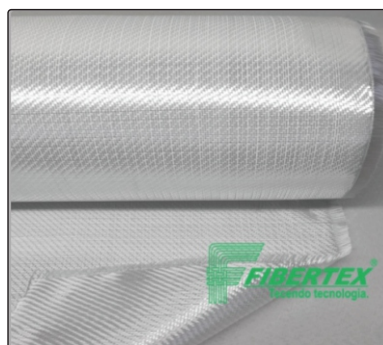
AF 0144 - 143g/m 2 | Twill 3x1
