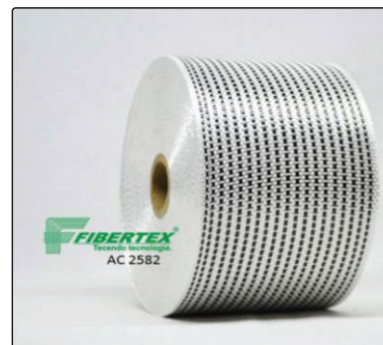
AC- 2582 Espessura: 0,25mm Largura: 80mm Comprimento do rolo: 50m
