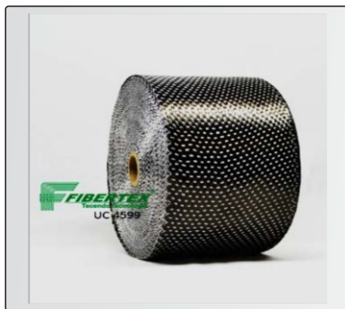
UC - 4599 Espessura: 0,45mm Largura: 100mm Comprimento do rolo: 50m
