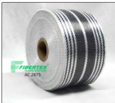
AC- 2875 Espessura: 0,25mm Largura: 75mm Comprimento do rolo: 50m
