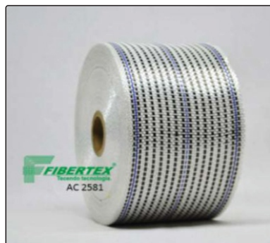
AC- 2581 Blue Espessura: 0,25mm Largura: 80mm Comprimento do rolo: 50m
