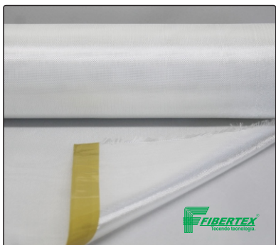
AF 0125 - 122g/m 2 | Screen 1x1
