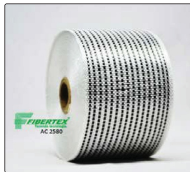
AC- 2580 Espessura: 0,25mm Width: 80mm Length: 50m
