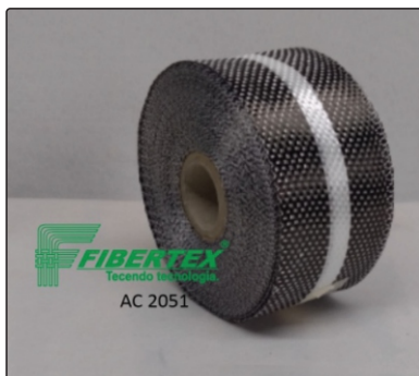
AC- 2051 Espessura: 0,20mm Width: 50mm Length: 50m
