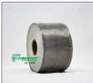
UC - 2950 Espessura: 0,29mm Largura: 50mm Comprimento do rolo: 50m
